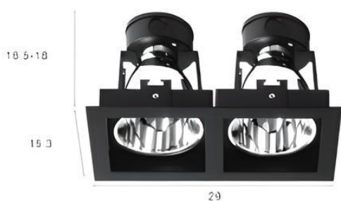
VL-6-B-668 E27 x 2 ⌀ 14 x 27.3 cm.
