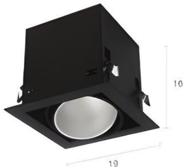
VL-6-B-671 E27 (PAR30) x 1 ⌀ 17.5 x 17.5 cm.
